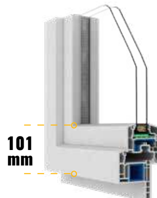
Variante DPP-70R35 avec ouvrant réduit
