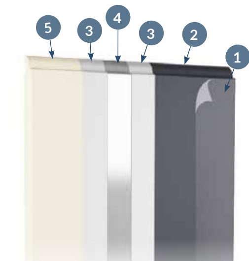
1. Film de protection | 2. Revêtement organique | 3. Galvan | 4. Acier | 5. Mousse polyuréthane
